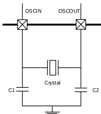
图5-7. HXTAL时钟源
