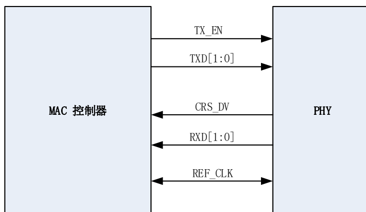
图 22-5. 精简媒体独立接口(RMII)信号线
