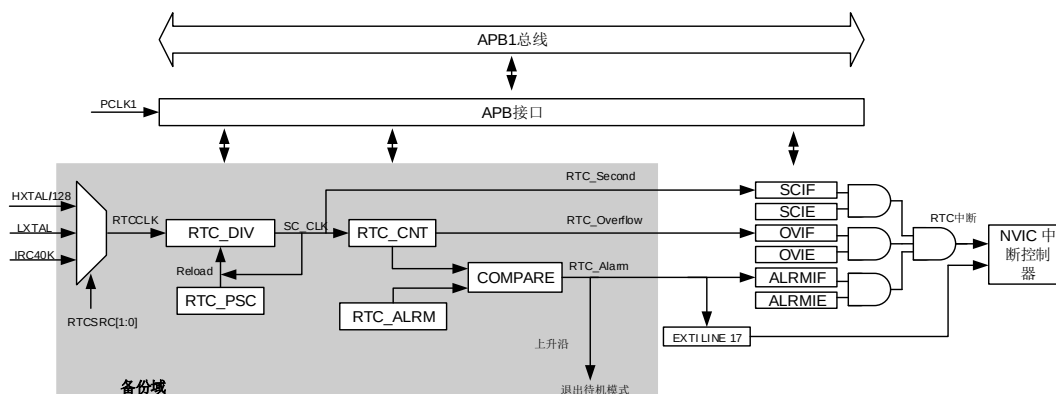
图 14-1. RTC 框图
