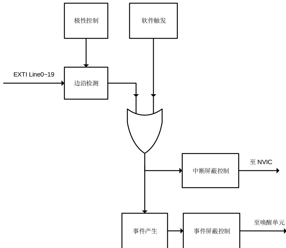
图 6-1. EXTI 框图
