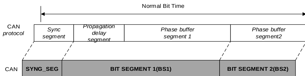
图 21-11. 位时序
