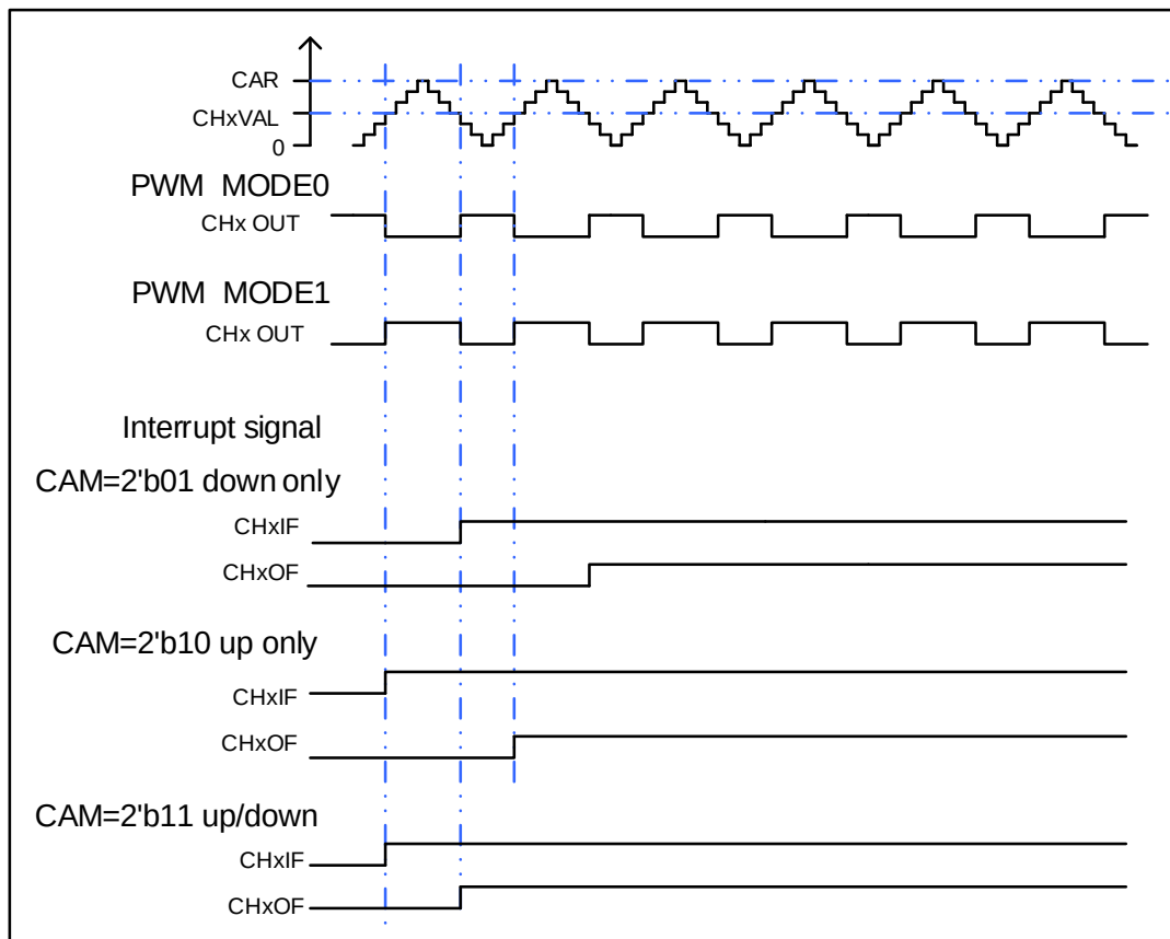
图 15-46. CAPWM 时序图
