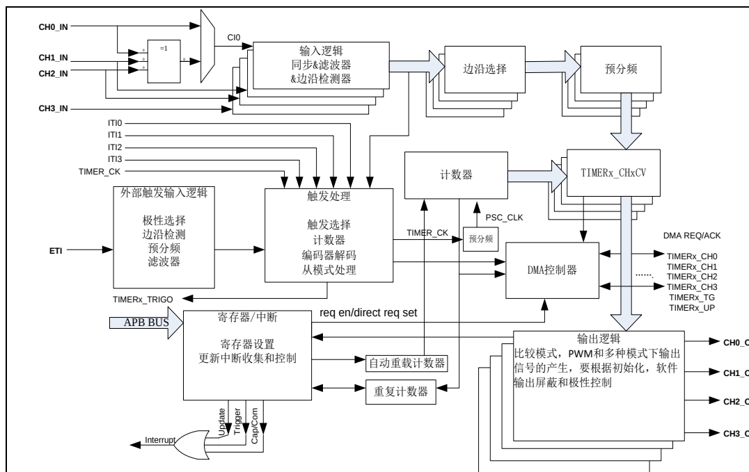
图 15-34. 通用定时器 L0 结构框图
