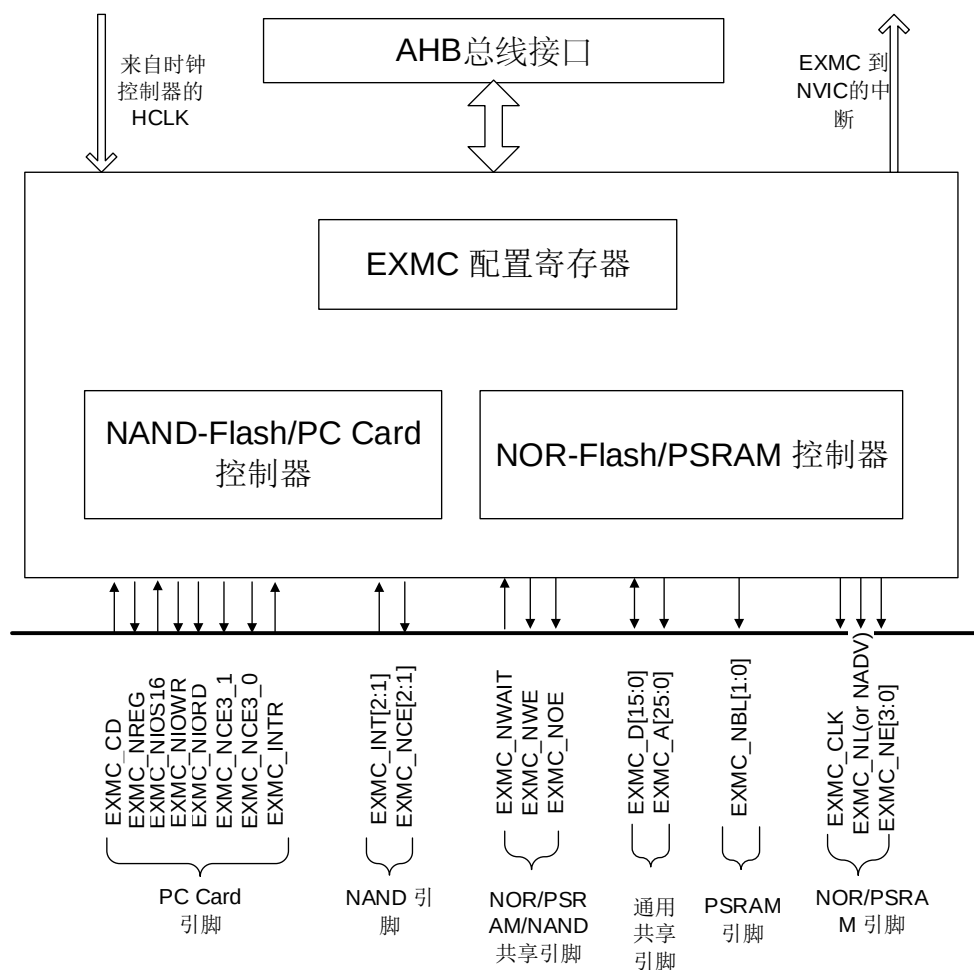
图 20-1. 系统架构
