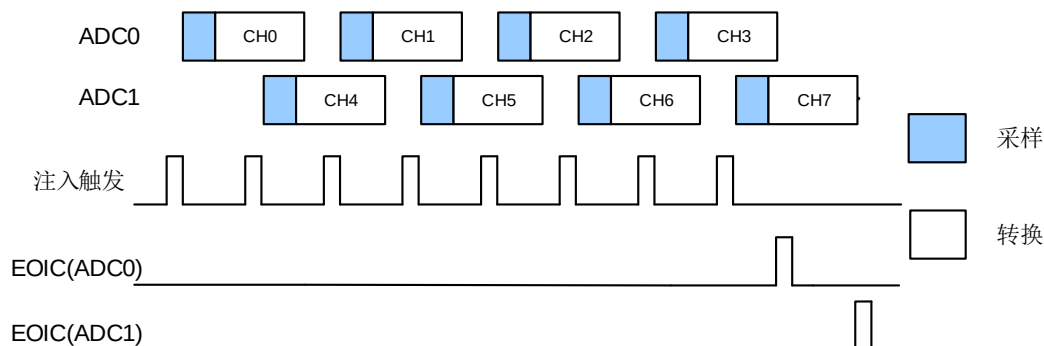
图 11-16. 交替触发: 中断模式下注入通道组
