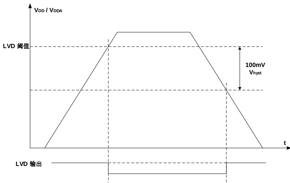
图3-3. LVD阈值波形图
