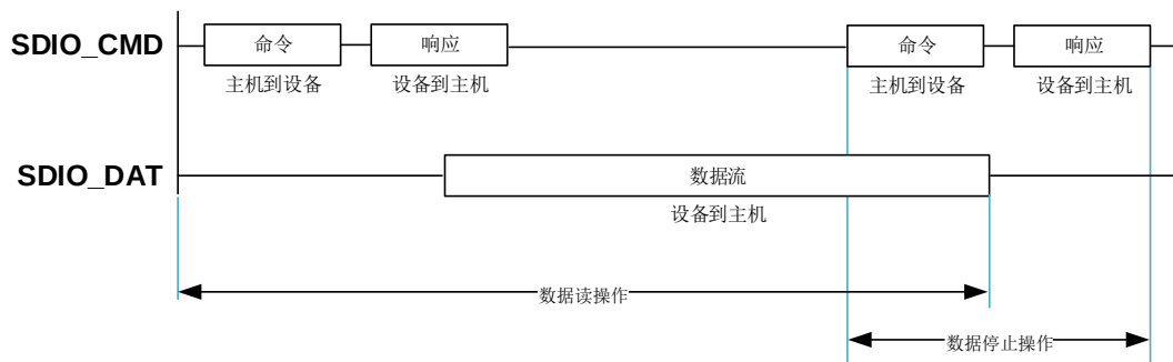
图 19-4. SDIO 数据流读操作
