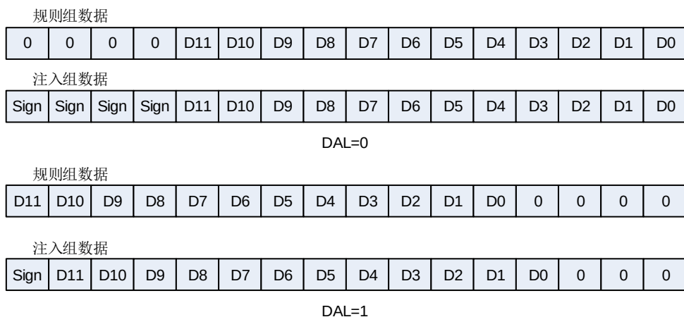
图 11-9. 12 位数据对齐
