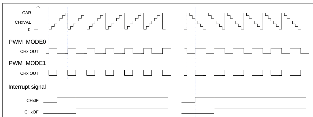
图 15-16. EAPWM 时序图
