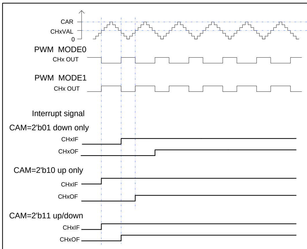
图 15-17. CAPWM 时序图
