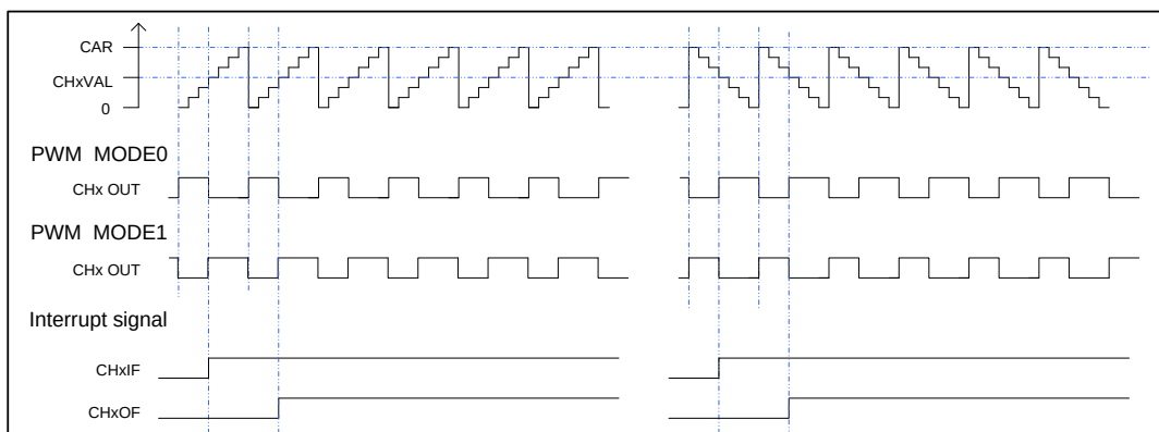
图 15-45. EAPWM 时序图
