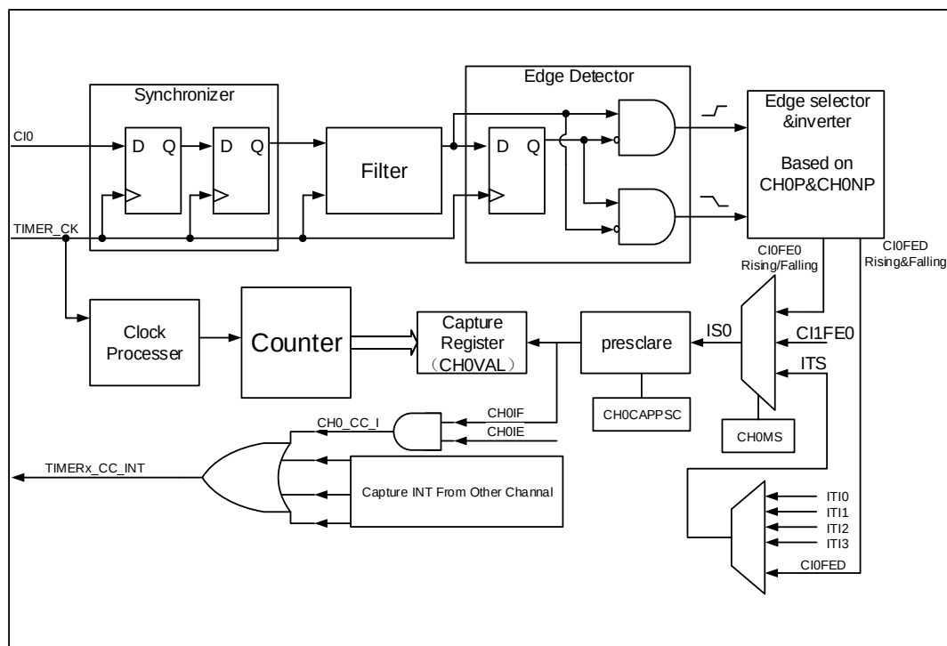
图 15-78. 输入捕获逻辑
