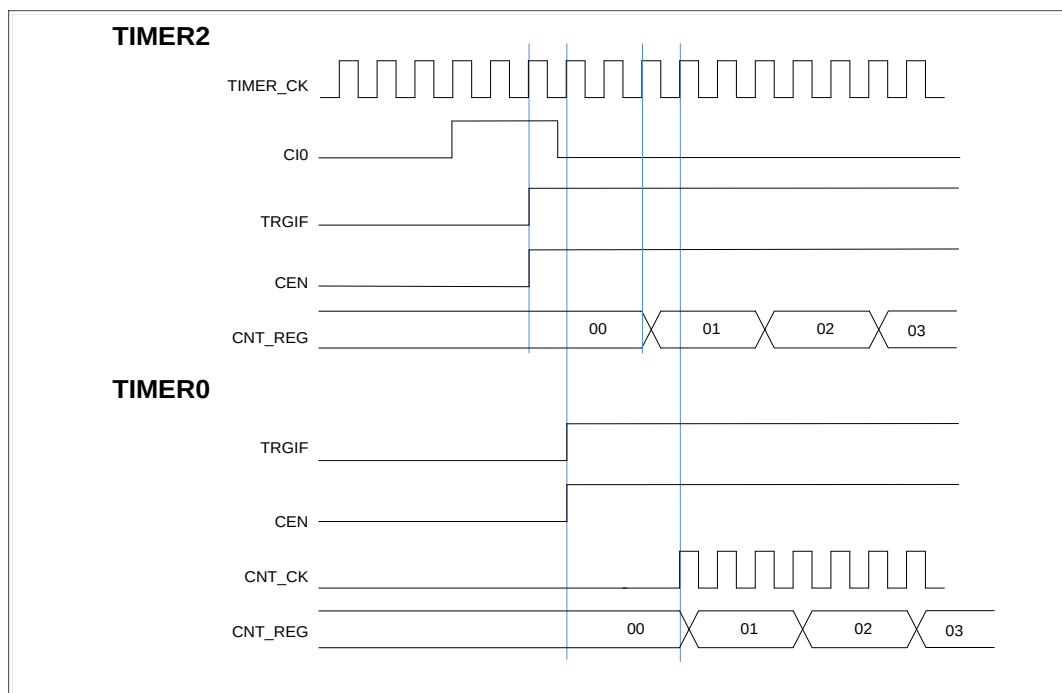
图 15-33. 用定时器 2 的 CI0 输入来触发定时器 0 和定时器 2
