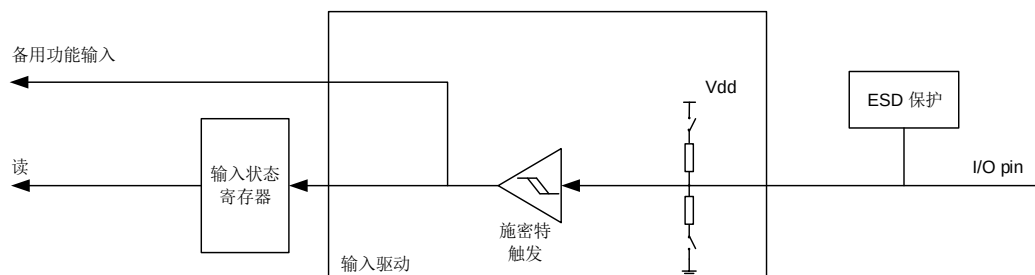
图 7-2. 输入配置
