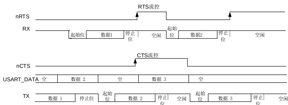
图 16-8. 硬件流控制
