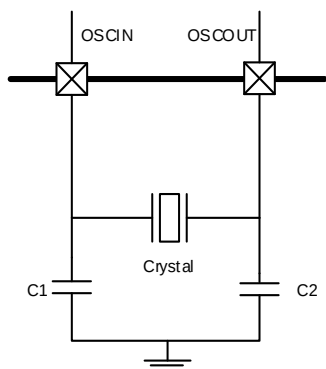
图5-3. HXTAL时钟源
