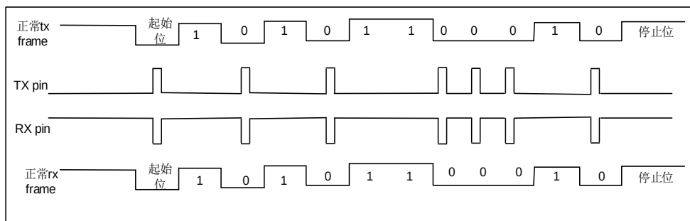
图 16-14. IrDA 数据调制
