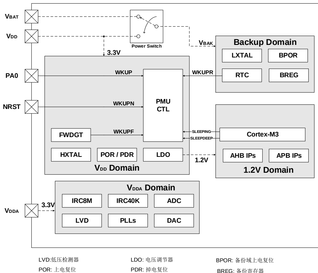
图3-1. 电源域概览
