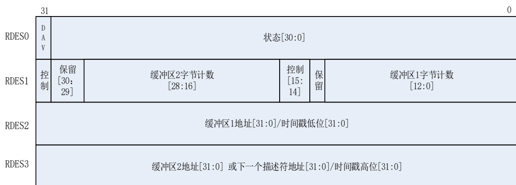
图 22-10. 接收描述符
