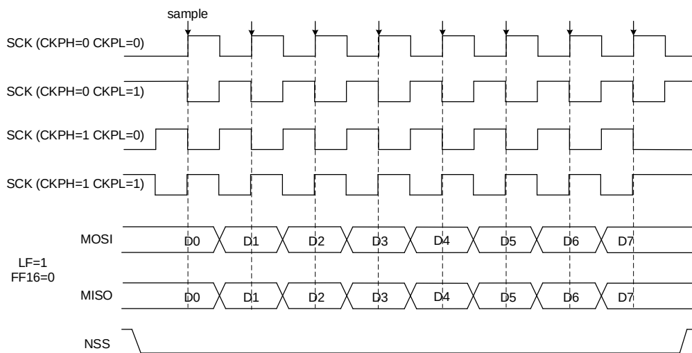
图 18-2. 常规模式下的 SPI 时序图
