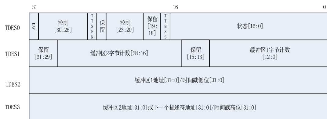
图 22-9. 发送描述符
